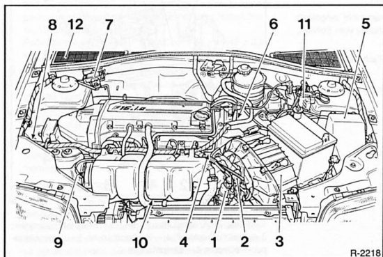
Motorraum-Übersicht: 16-Ventil-Motor
