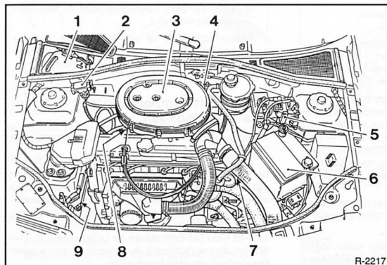
Motorraum-Übersicht: 16-Ventil-Motor
